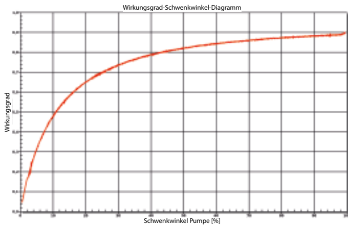
» Abb. 3: Wirkungsgrad-Schwenkwinkel-Diagramm
