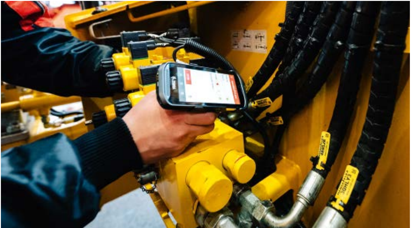
» Das Label an den Leitungen enthält den X-CODE nicht nur schriftlich, sondern auch digital auf einem RFID-Chip mit HF-Technologie. Diese erlaubt nur kurze Auslesedistanzen von wenigen Zentimetern. » The label on the hose not only contains the X-CODE in writing, but also digitally on an RFID chip. This allows only short read-out distances of a few centimetres.
