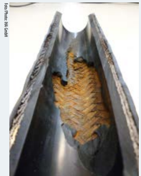
» Abb. 4: Folge: Auswaschungen und Durchschüsse
